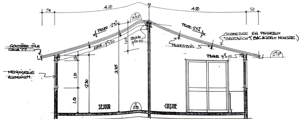
COUPE A.A
