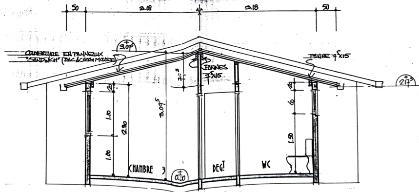
COUPE B.B
